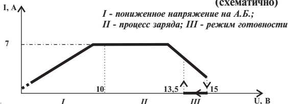
Вольт-Амперная характеристика работы Вымпел-150 (схематично)
